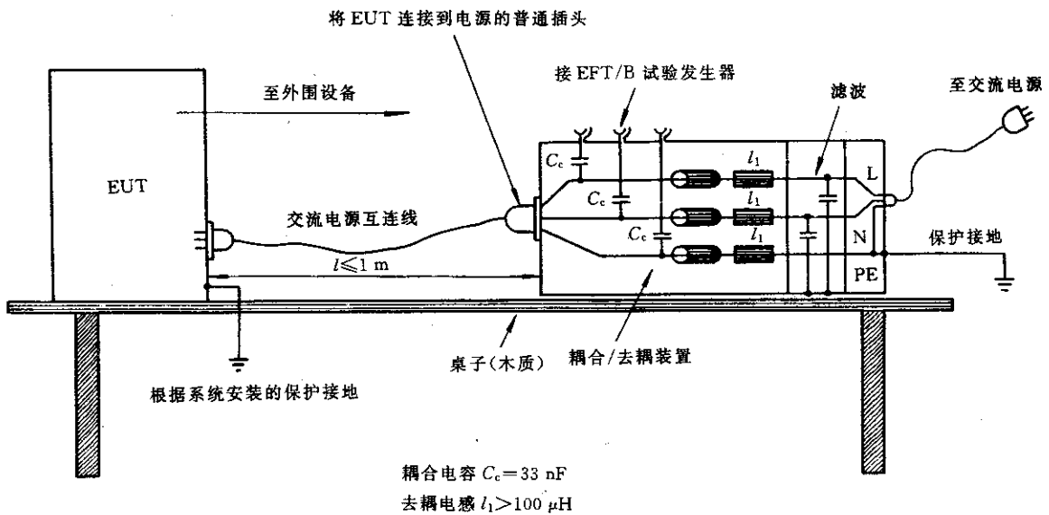
图 11 非固定式受试设备交流电源端口和保护接地端子安装后试验示例
