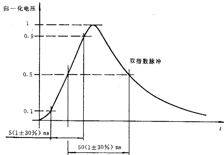
图 3 接 50 \Omega 负载时单个脉冲的波形
