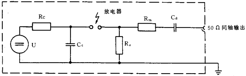
图 1 快速瞬变脉冲群发生器电路简图
