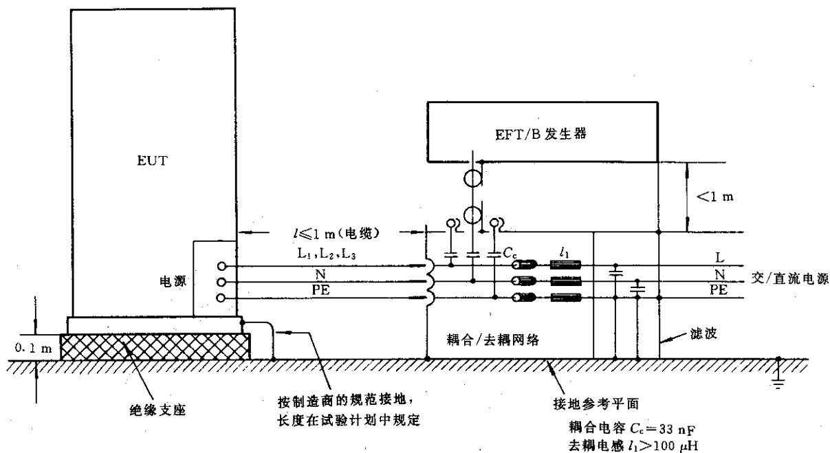
图 8 用于实验室试验的试验电压直接耦合到交流/直流电源端口/端子的试验配置示例
